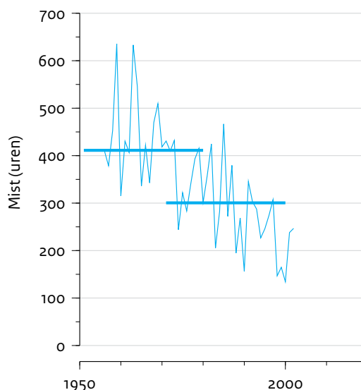
FIGUUR 13 Jaarlijks aantal uren mist (zicht minder dan 1 km) in Nederland.
