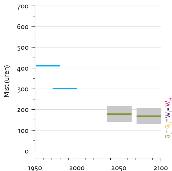
FIGUUR 14 Mistklimaat (zicht minder dan 1 km) in Nederland: waarnemingen en berekeningen volgens de KNMI'14-scenario's. Aan het einde van de visuele waarneemreeks in 2002 was het jaarlijks aantal uren mist al afgenomen tot ongeveer 200 uur.
